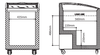
F14 Internal Dimensions
